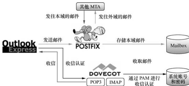
图 15-3 电子邮件系统的工作流程
